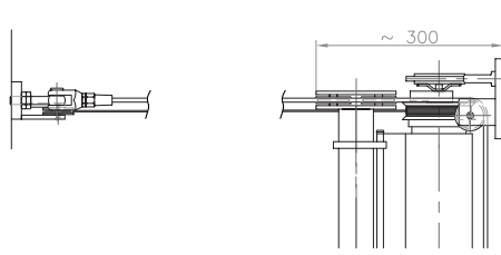
Umlenkung der Zugseile Tragsailanbindung
