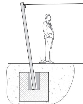
BS 3: Stütze für Kocherfundament*
