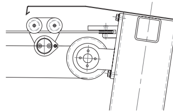
Wellenkonzole an der freistehenden Stütze
