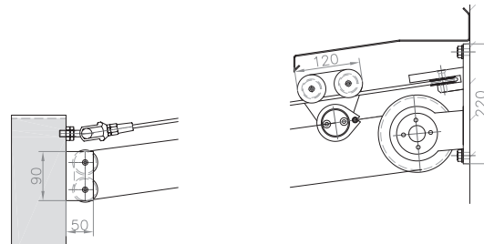
Umlenkung der Zugseile Tragsailanbindung
